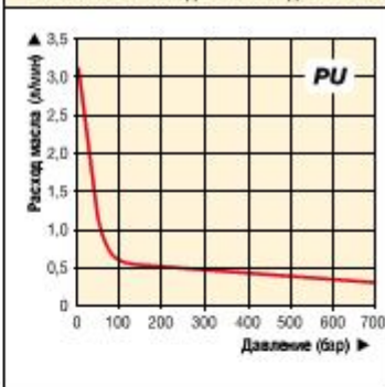
ЗАВИСИМОСТЬ РАСХОДА МАСЛА ОТ ДАВЛЕНИЯ
