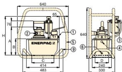
Насосы серии ZA4 с 4 – 6,6-литровыми резервуарами
