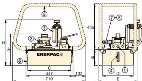
Насосы серии ZA4 с 10, 20 и 40-литровыми резервуарами
